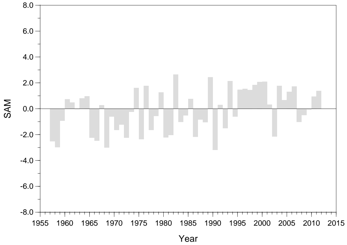
SAM Index: Autumn (MAM)
